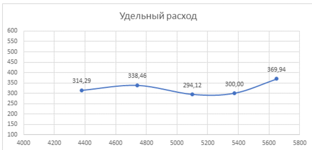
Рис 3. Удельный расход топлива DM-96 г/л.с. ч. с пропеллером 26x12.
