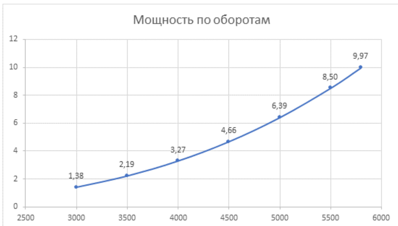
Рис 2. Мощность DM-96 по оборотам, л.с. с пропеллером 26x12.
